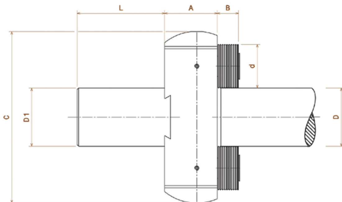
Tangonvetotyökalun rakennepiirros.
