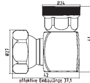
2-WV-1K Winkelstück elbow piece
