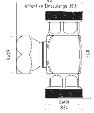
2-WV-2K T-Stück T-piece
