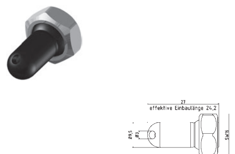
KU-1-DU-30 Kunststoff-Düse 30° Bohrung Ø 3 mm plastic nozzle 30° drill hole Ø 3 mm
