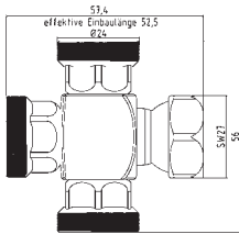
2-WV-3K Kreuz-Stück cross piece
