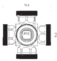
2-WV-4K Stern-Stück star piece
