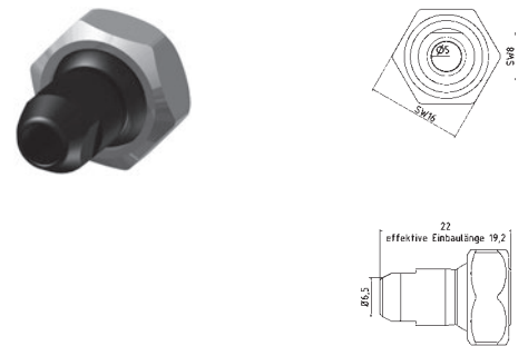
KU-1-DU-50 Kunststoff-Düse gerade Bohrung Ø 5,0 mm plastic nozzle straight Ø 5,0 mm
